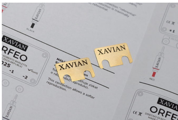
Orfeo有4种连接方式，其中2种连接方式需要借助厂家随产品所附的连接片
